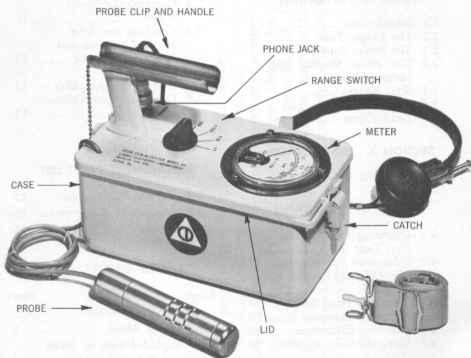
Fig. 1 — Lionel CD V-700 Survey Meter
