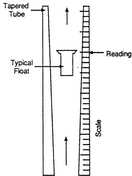
Figure 5.1. Rotameter
